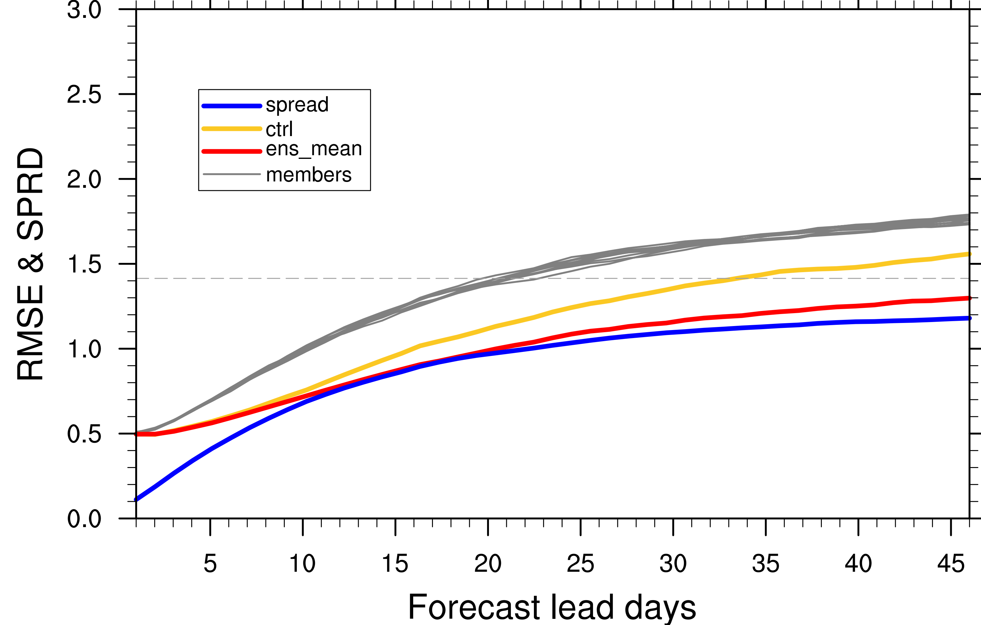
(b) ECMWF
