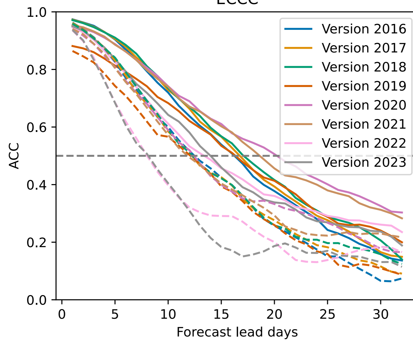
ECCC
