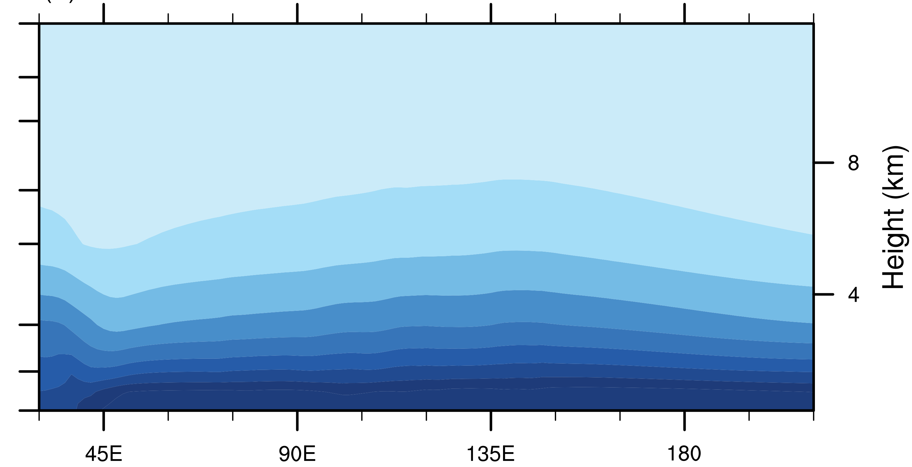
(b) Pred
