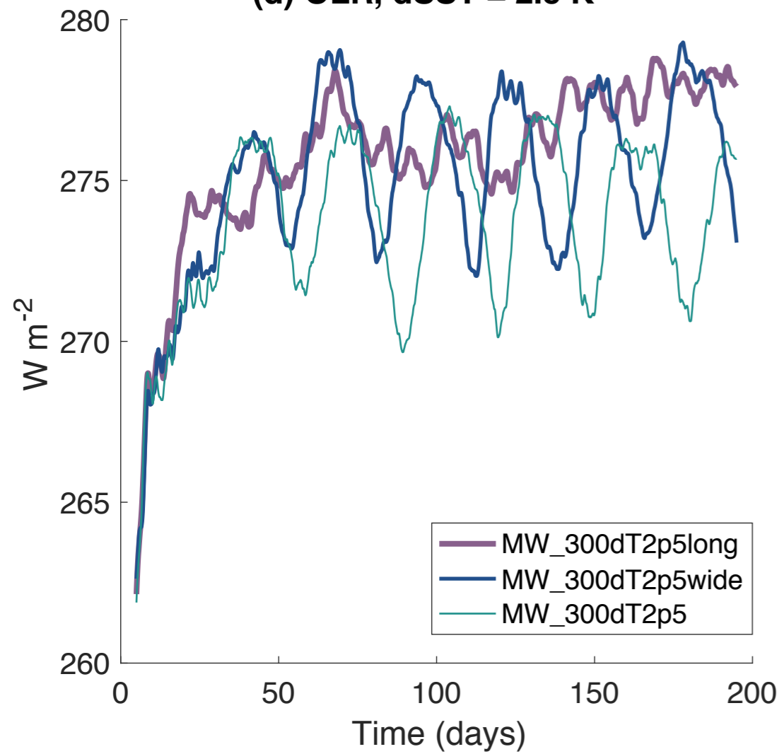
(d) OLR, dSST = 2.5 K
