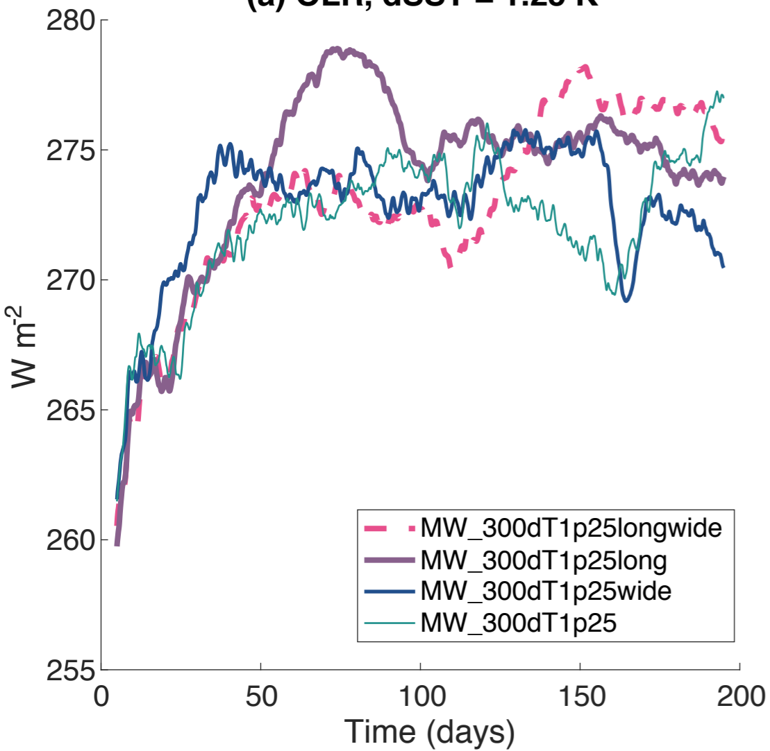
(a) OLR, dSST = 1.25 K
