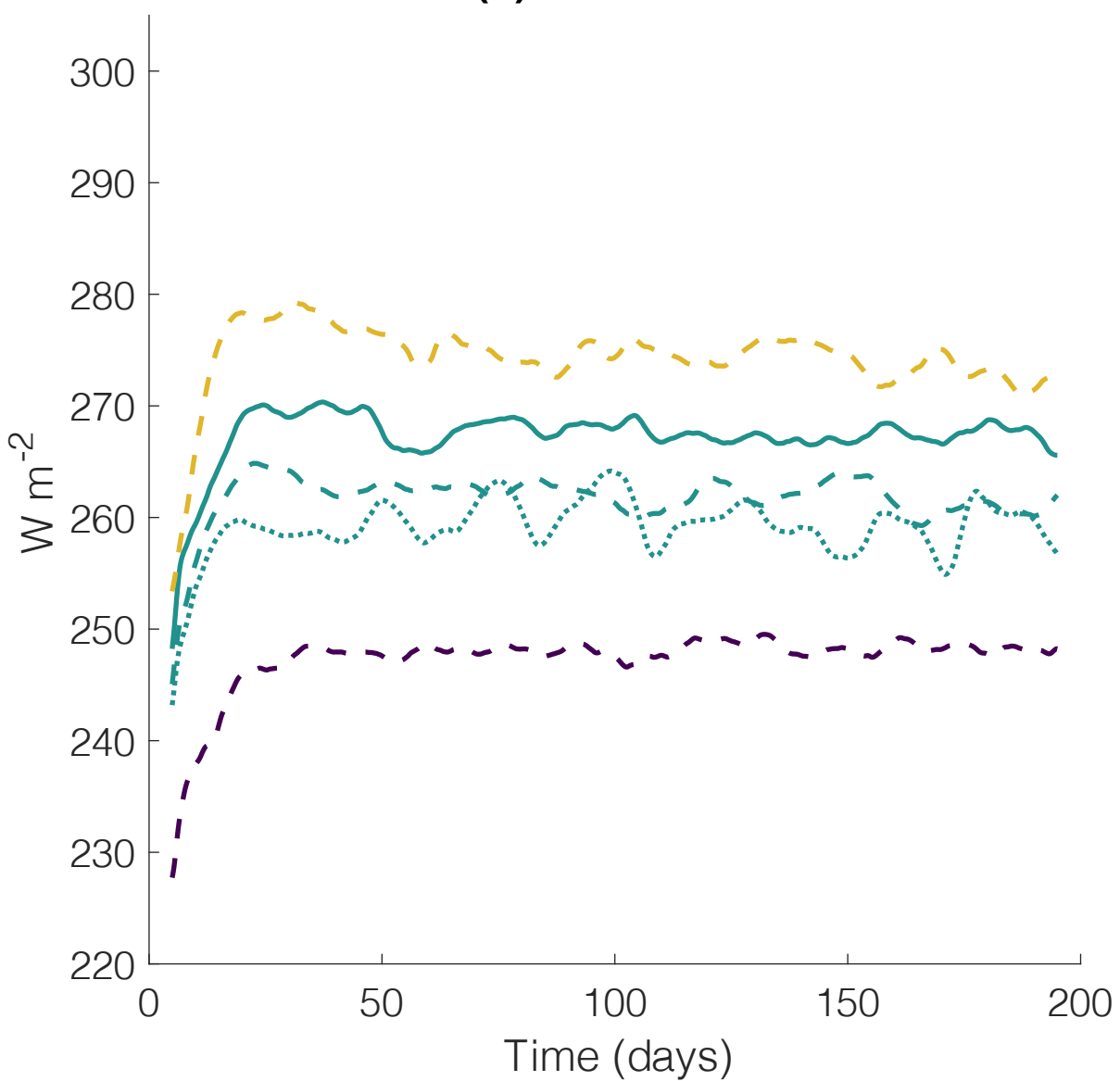
(d) CAM: OLR
