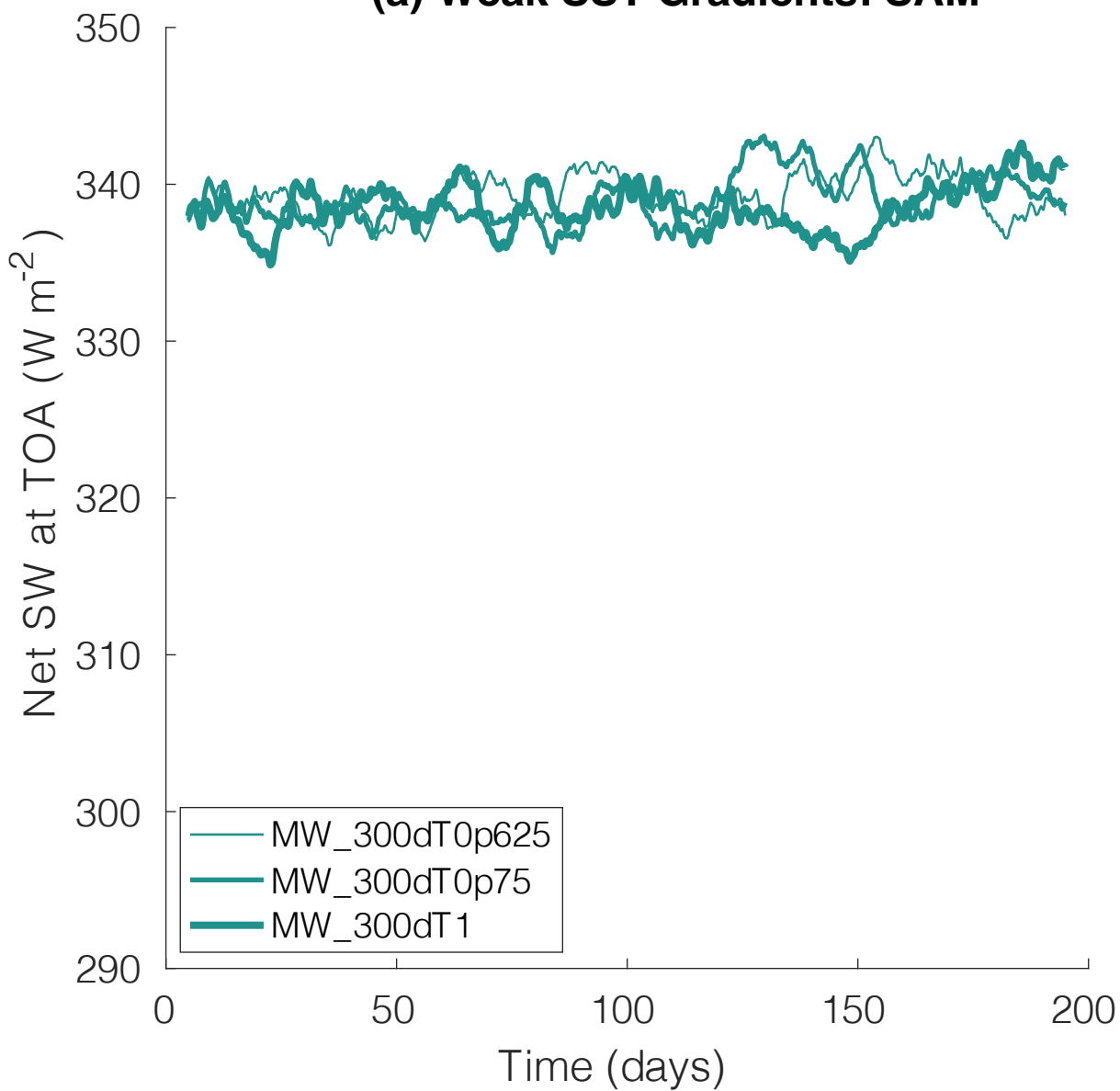
(d) Weak SST Gradients: CAM
