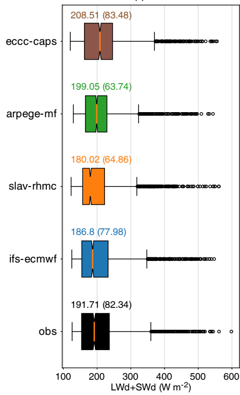
Radiation (f) Tiksi
