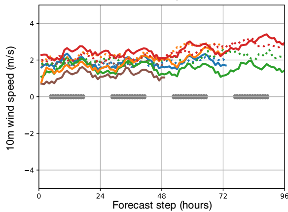
(f) Ny-Alesund
