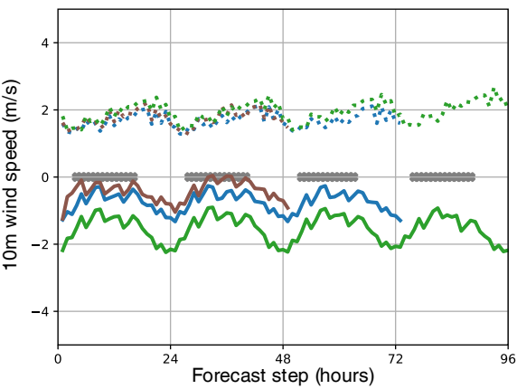
(c) Sodankyla
