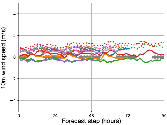
(e) Tiksi
