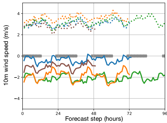
(d) Utqiagvik
