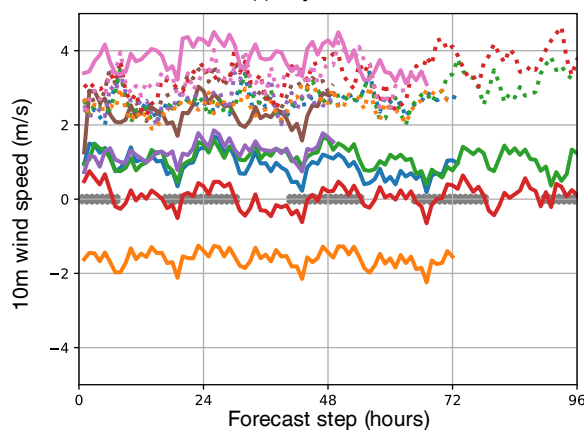
(f) Ny-Alesund
