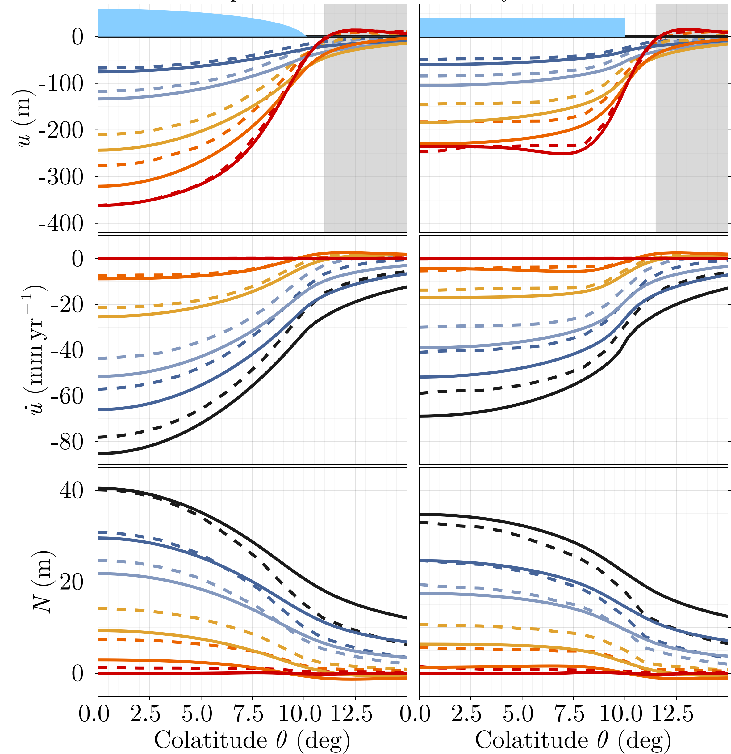
Cap load
