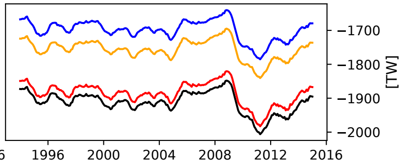
(d) Drake heat transports
