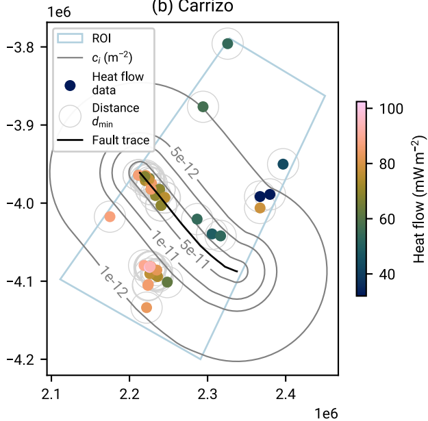
(b) Carrizo
