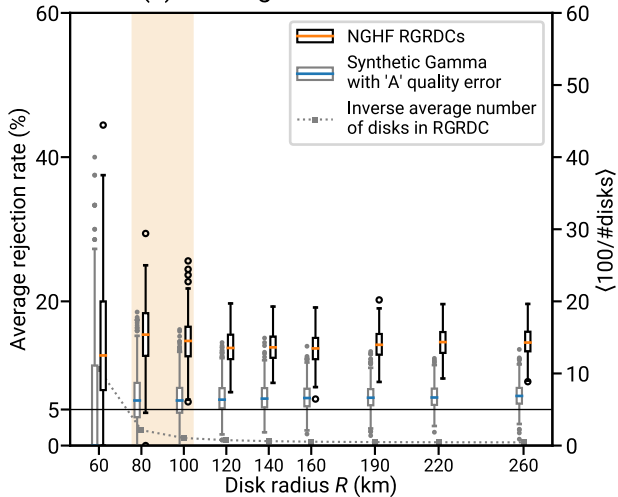
(a) Kolmogorov-Smirnov test
