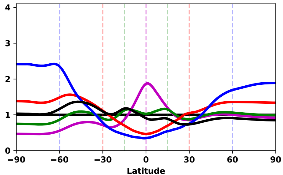
(d) CESM2 \Delta Ts (2050-2069)
