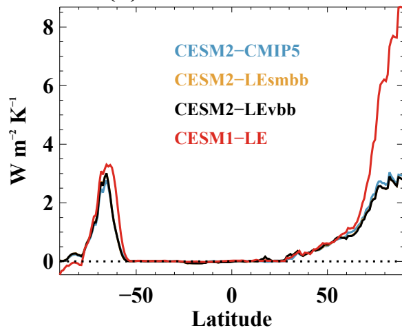
(b) 2080–2100 AlbFB
