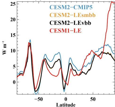
(d) Attribution 2080–2100 \Delta FSNT
