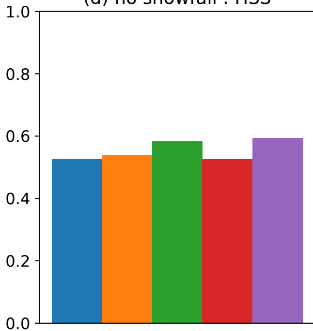
(d) no snowfall : HSS
