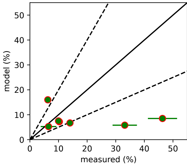
Hematite
