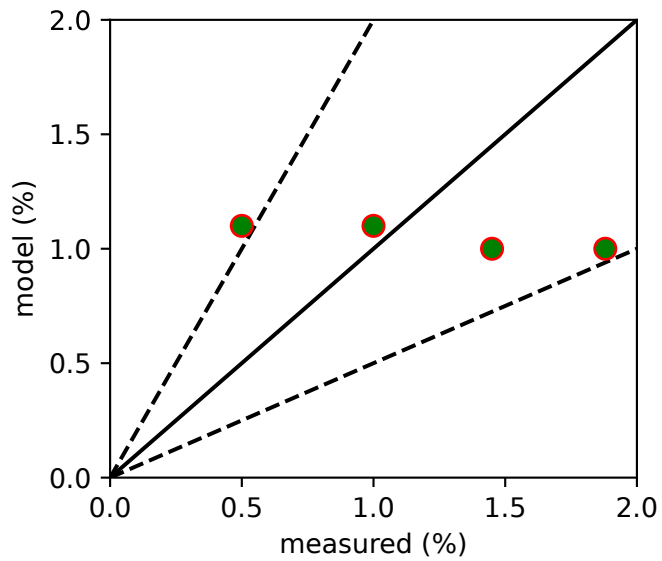
Hematite
