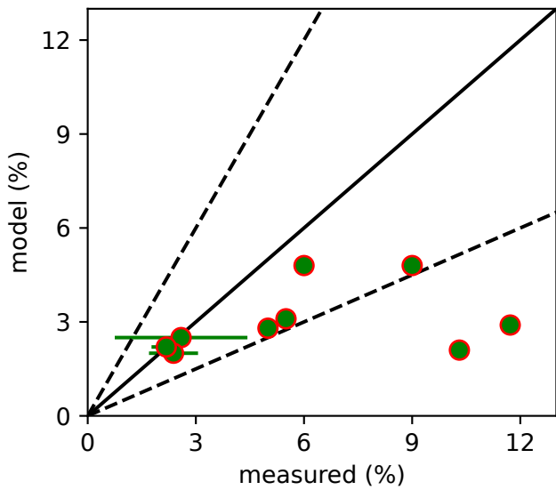
Calcite
