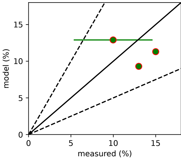
Calcite
