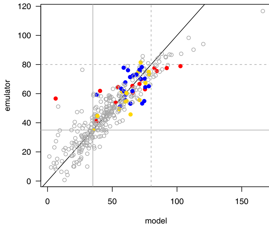
npp_nlim_Ind_sum
