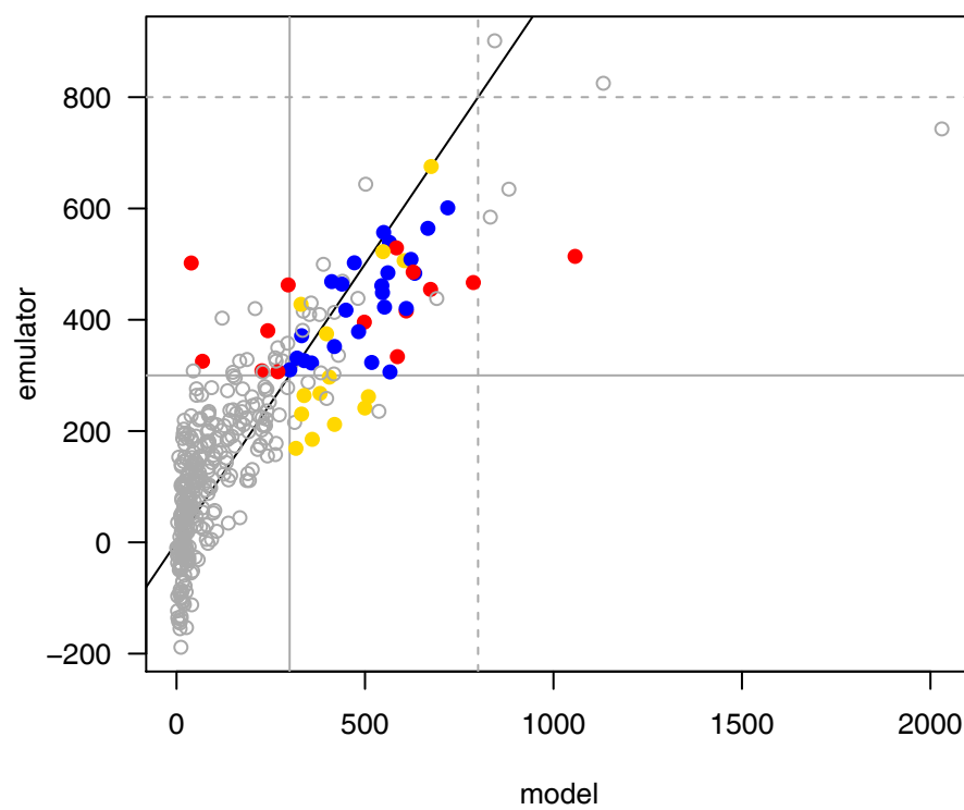
cVeg_Ind_sum
