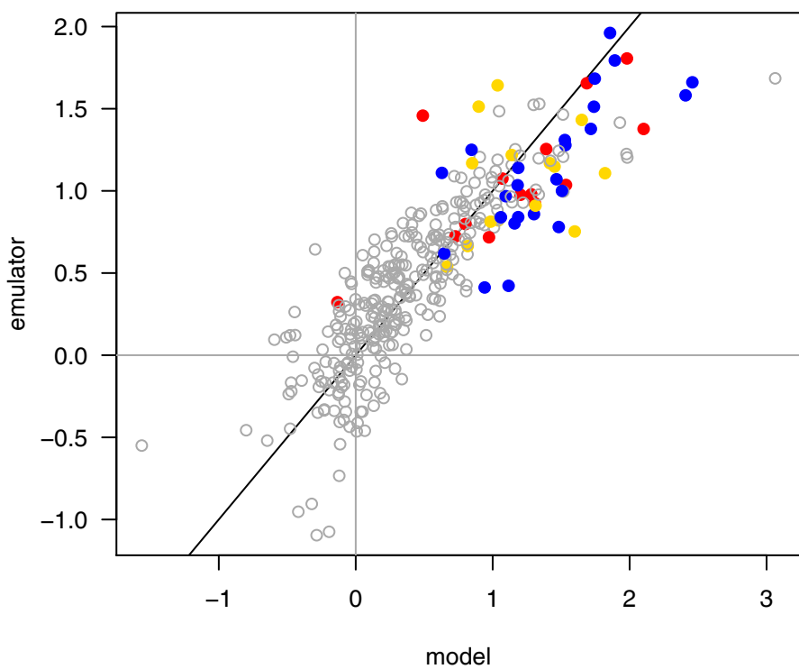
nbp_Ind_sum
