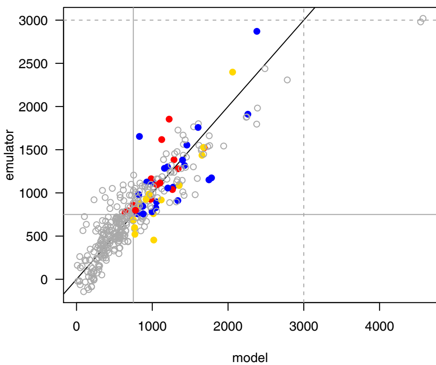
cSoil_Ind_sum
