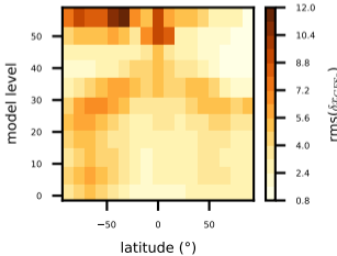
(d) gefs100 U (m/s)
