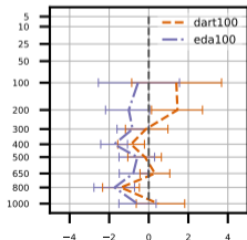
(d) V (m/s) at 1.0 d
