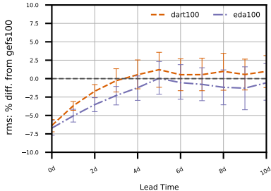
(d) V (m/s)
