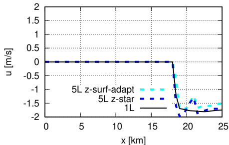
(d) channel x-velocity at t=21600.0 s
