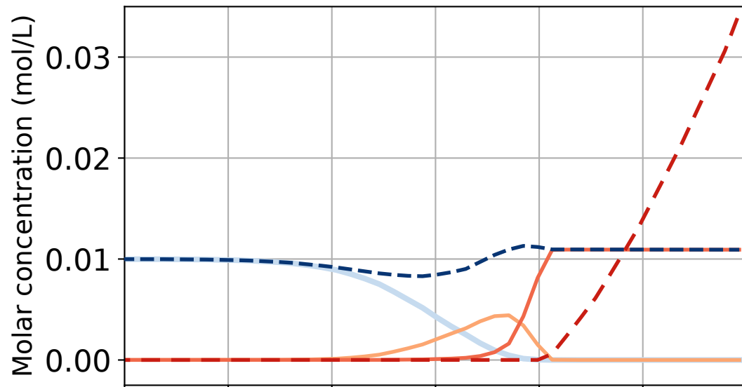
Nernst-Planck
