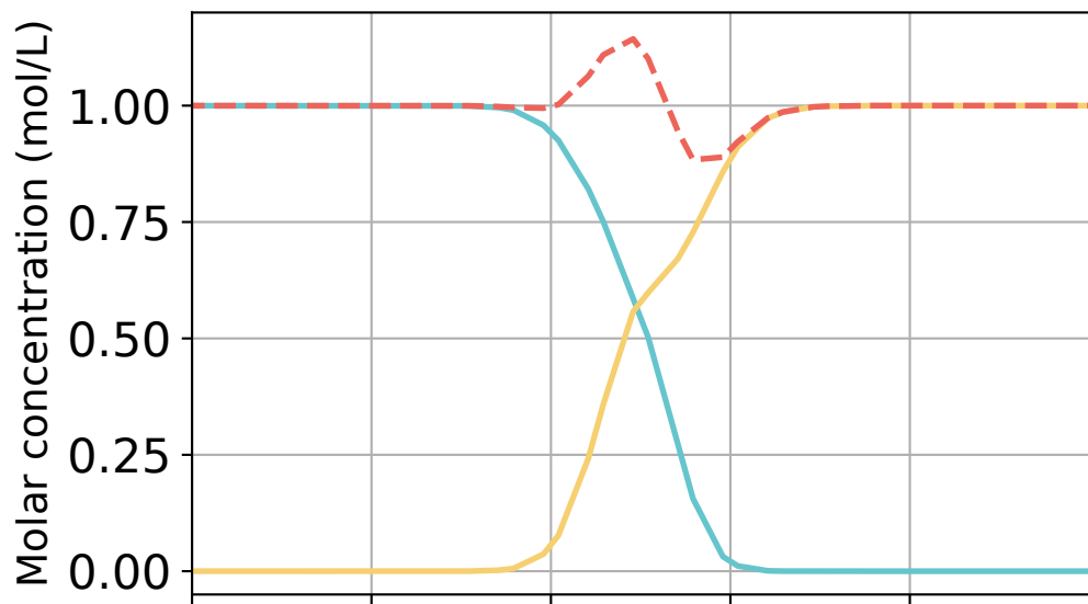
Nernst-Planck
