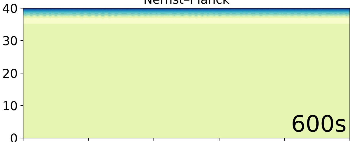
Nernst-Planck
