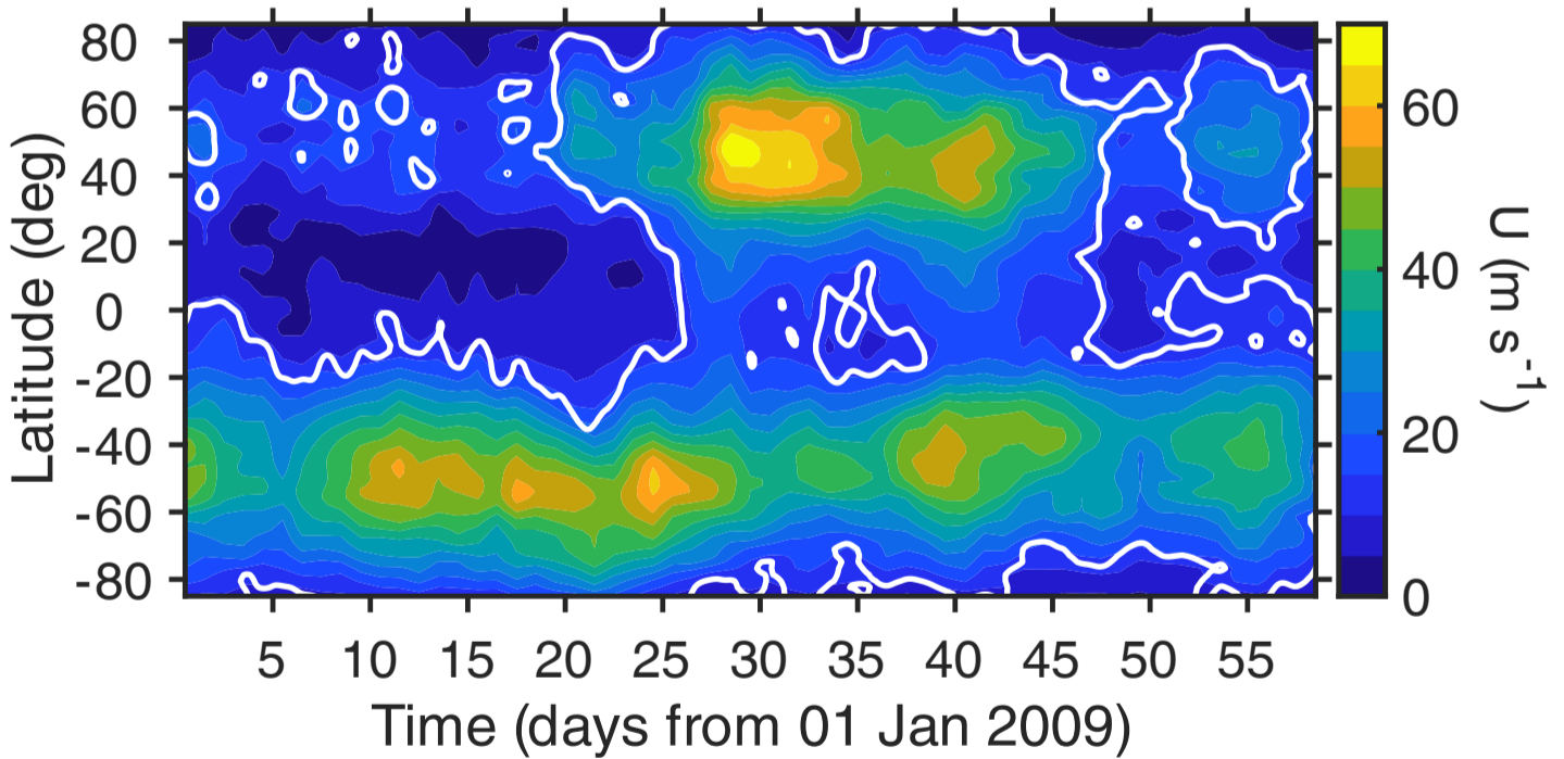
(d) Migrating diurnal tide at 95 km
