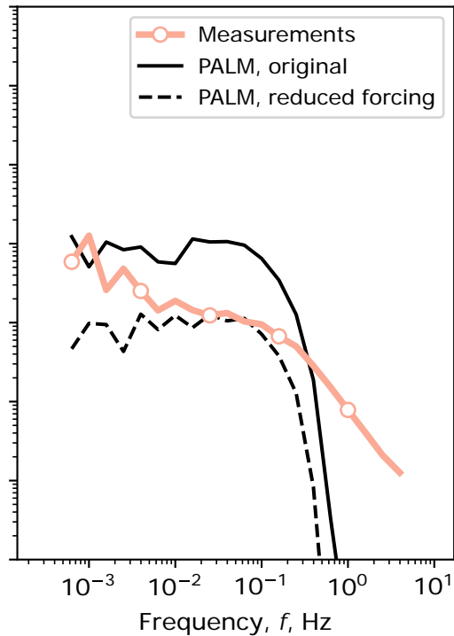
(b) w-spectra
