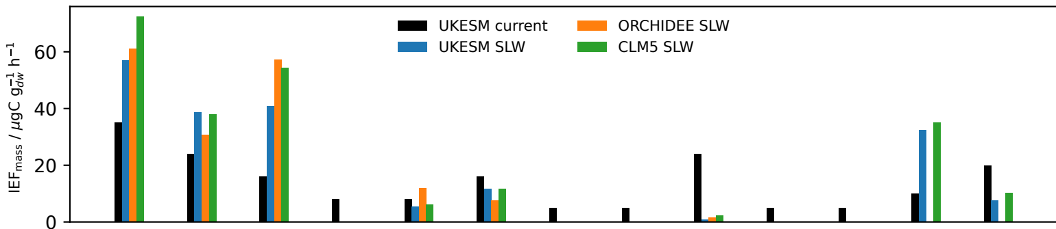
(a) IEF_{mass} on UKESM PFTs
