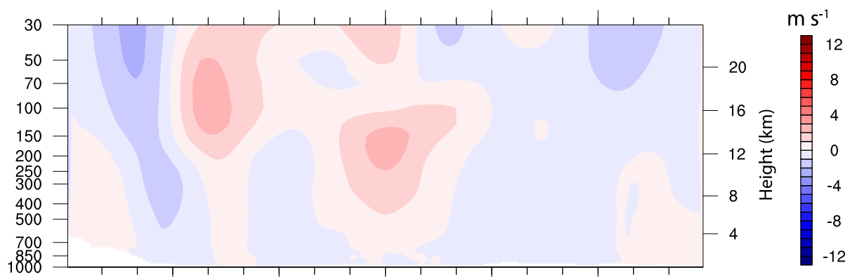
(d) [VR50-200] - [UR120]
