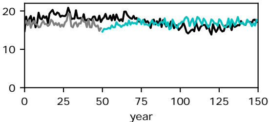
CESM2
