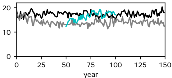
MPI-ESM1-2-HR
