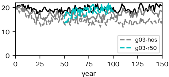
MPI-ESM1-2-LR
