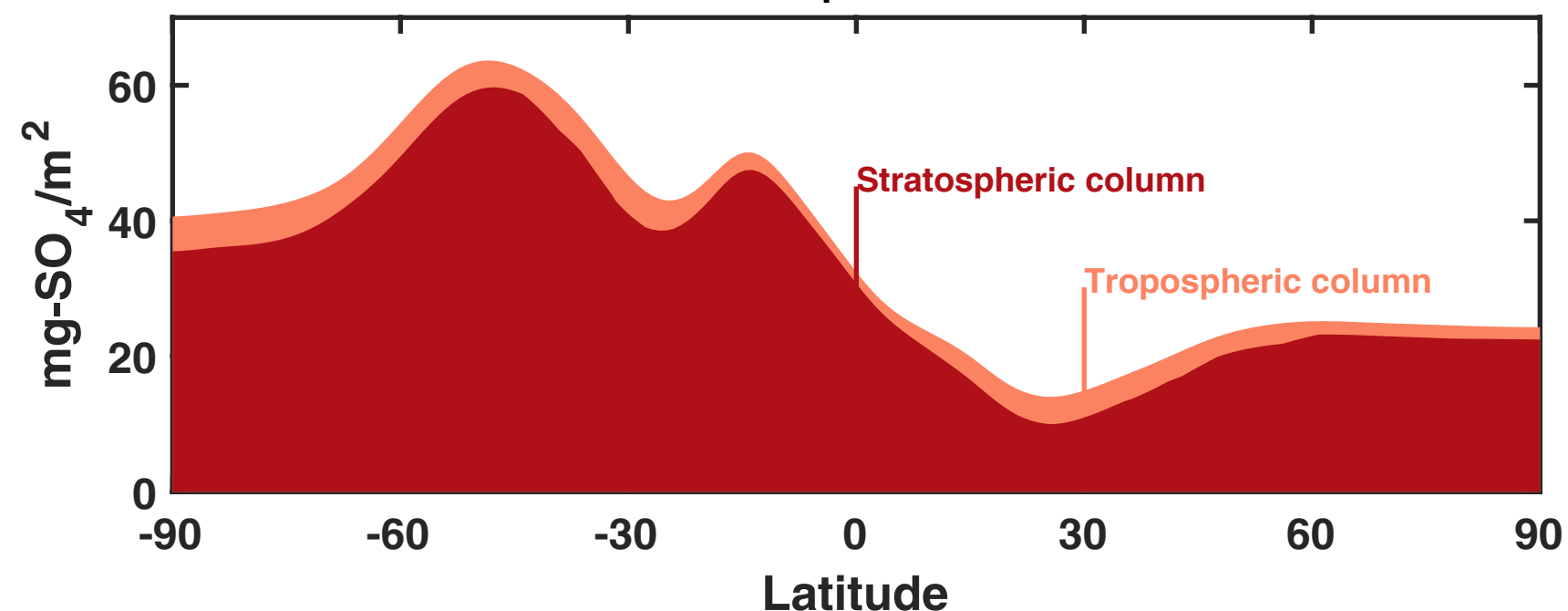
(d) Total column SO 4 increase [2050-2069]
