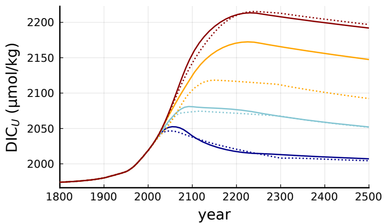
(c) Upper ocean layer DIC
