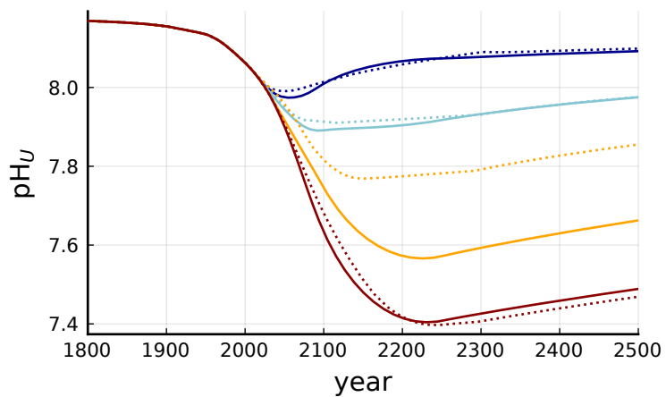
(d) Upper ocean layer pH
