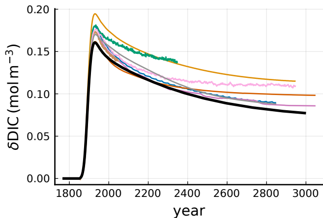
(d) Upper ocean layer DIC anomaly
