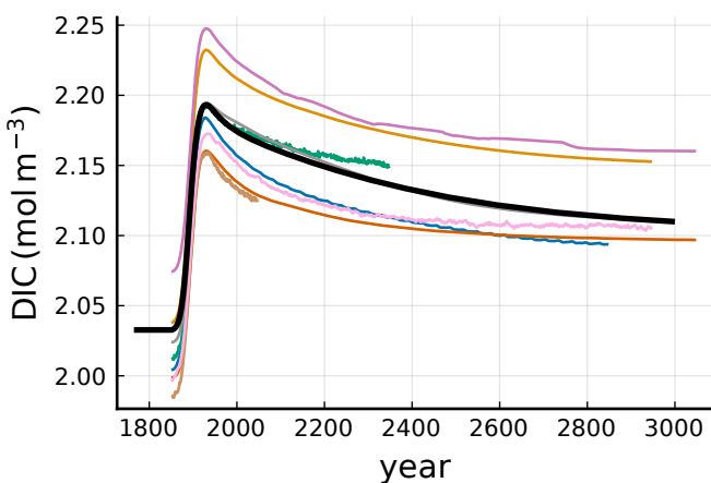
(c) Upper ocean layer DIC
