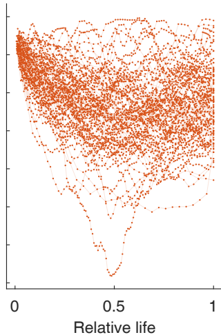
Synthetic (ERA-5)
