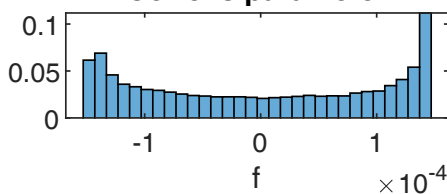
Coriolis parameter
