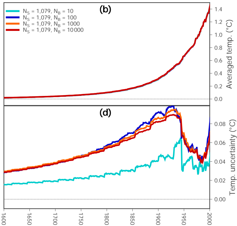
Xibalbá Dataset
