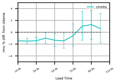
(d) V
