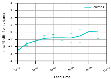
(b) Qv01to30
