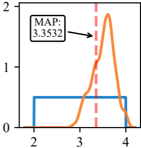
Smagorinsky visc. PDF
