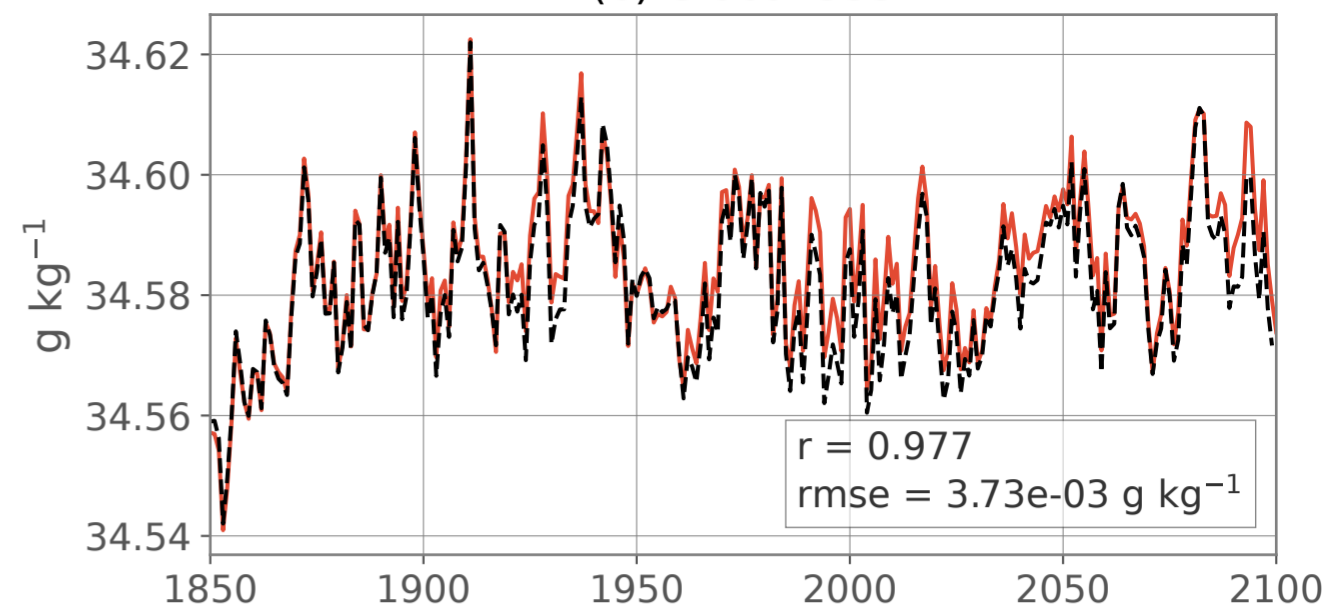
(d) Global salinity at 500 m
