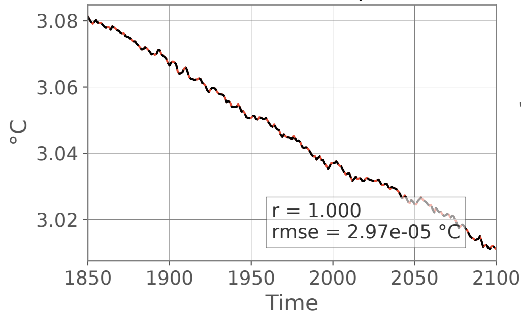
(d) Global mean temperature
