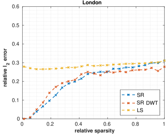
(b) \frac{m}{n} \approx 75\%
