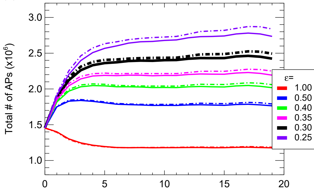
(a) CLaMS-2.0, Start: 01.01.2017
