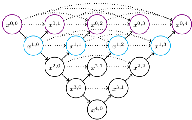
(b) U-Net++
