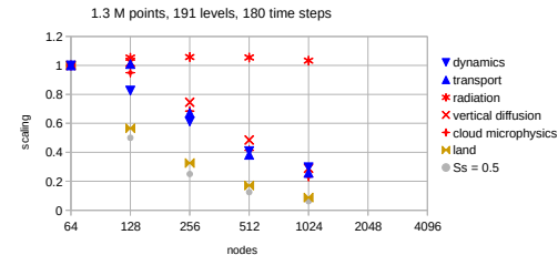
(d) Juwels-Booster: Cumulative strong scaling of component
