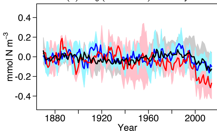
(d) NO 3 (0 – 100 m) anomaly
