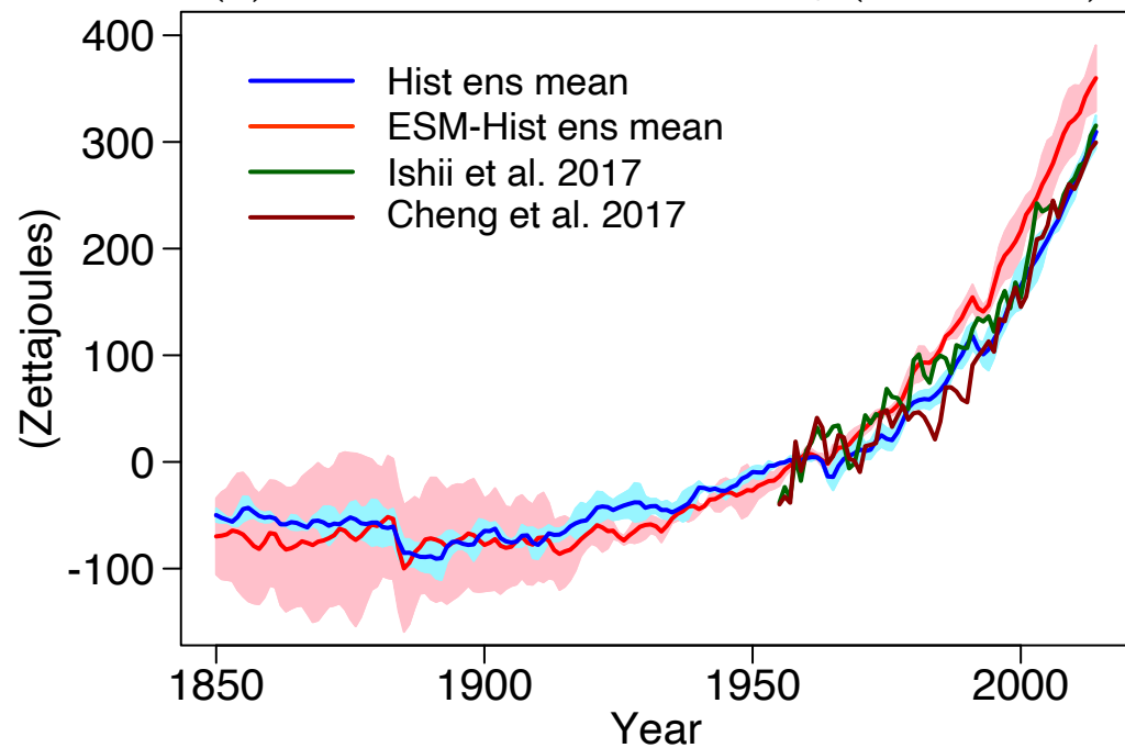
(d) Ocean heat content anomaly (0 – 2000 m)
