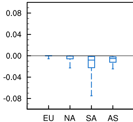
(b) OH
