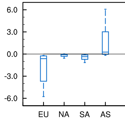
(f) flxn( O_3^{tra} )
