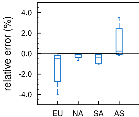
(d) O_3^{tra}
