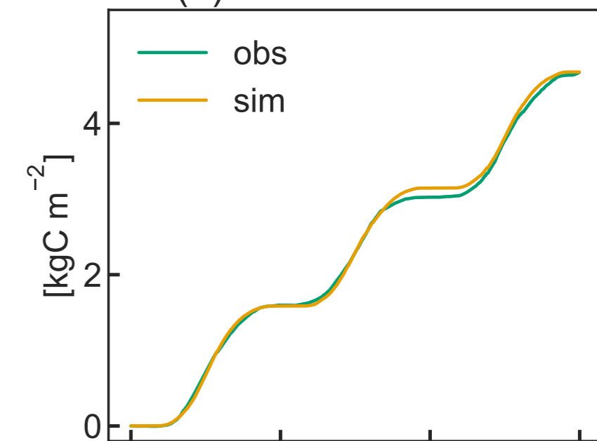
(d) Cumulative NEE
