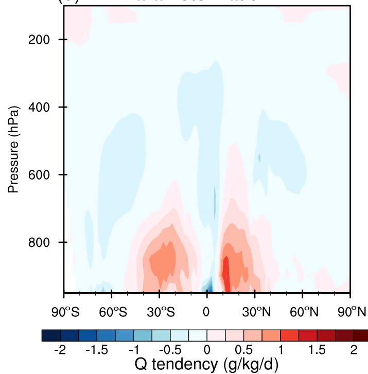
(d) NN-Parameterization
