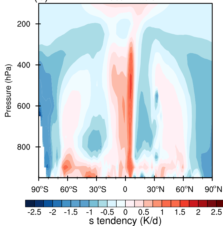
(d) NN-Parameterization
