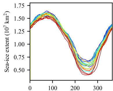
(d) SH MPAS-Seaice extent
