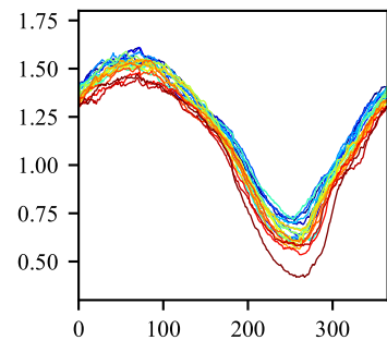
(f) SH SSMI extent
