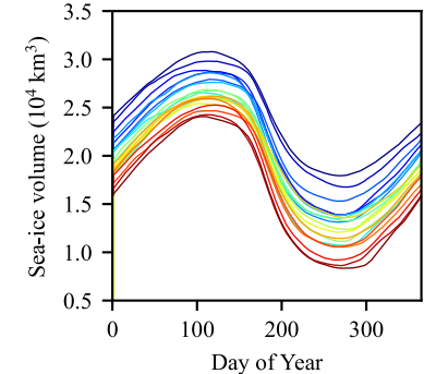
(g) NH MPAS-Seaice volume
